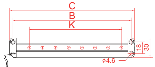
圖(1) 標準型 直接出線 雙孔固定
