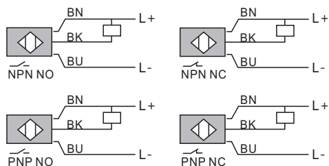
芯線顏色 BN棕色 BU藍色 BK黑色
