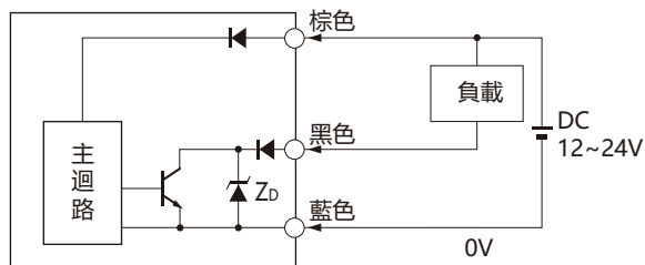
NPN
